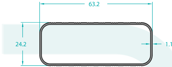
15139 0,466 Kg/m
