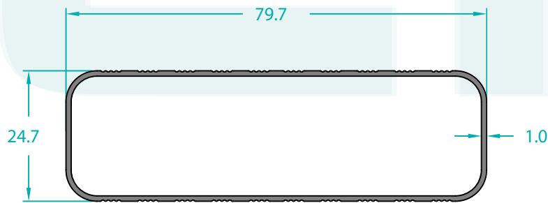
15137 0,509 Kg/m
