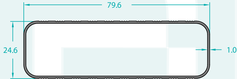
15136 0,482 Kg/m
